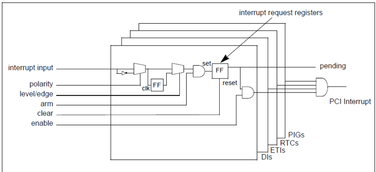
図3-1 割込み処理ロジック
