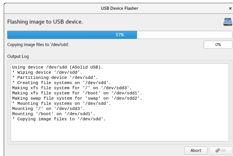
図1-59 進行中のフラッシュ・コピー
