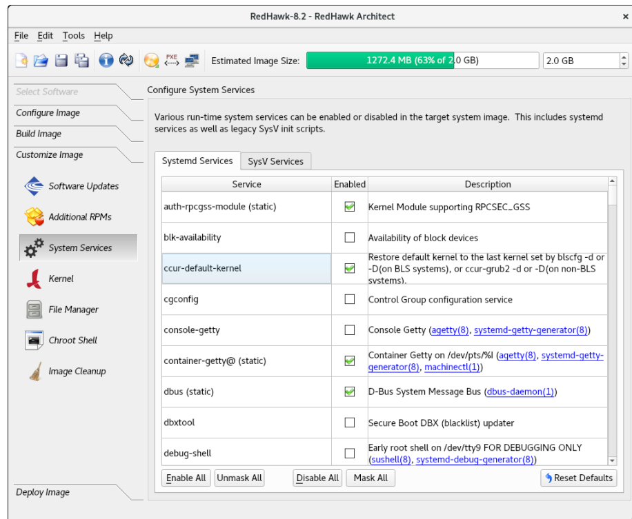
図1-46 System Servicesページ
