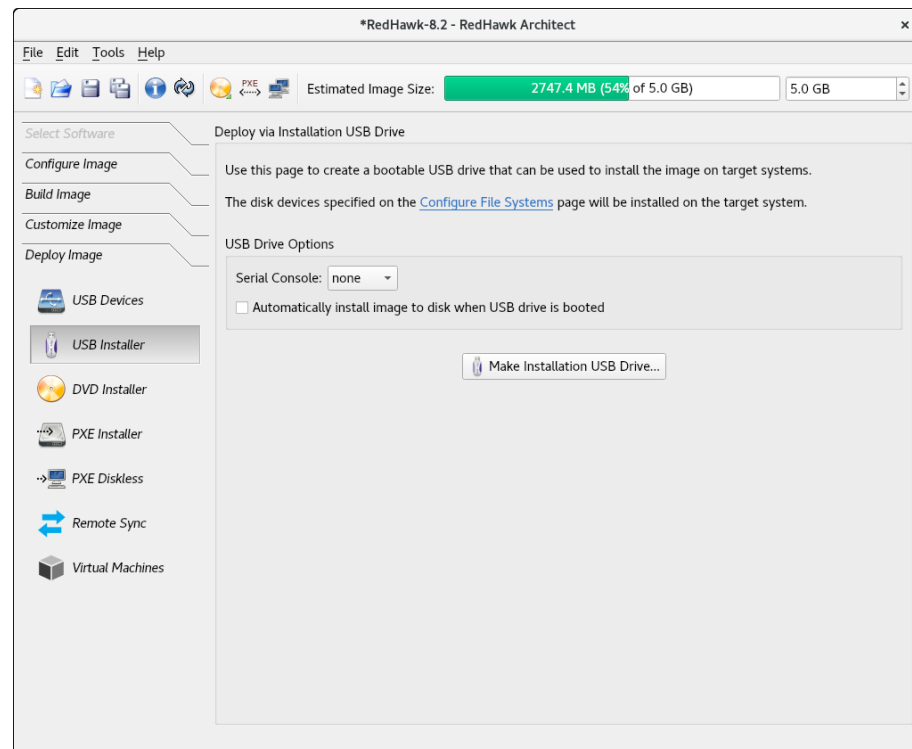
図1-62 Deploy via Installation USB Driveページ
