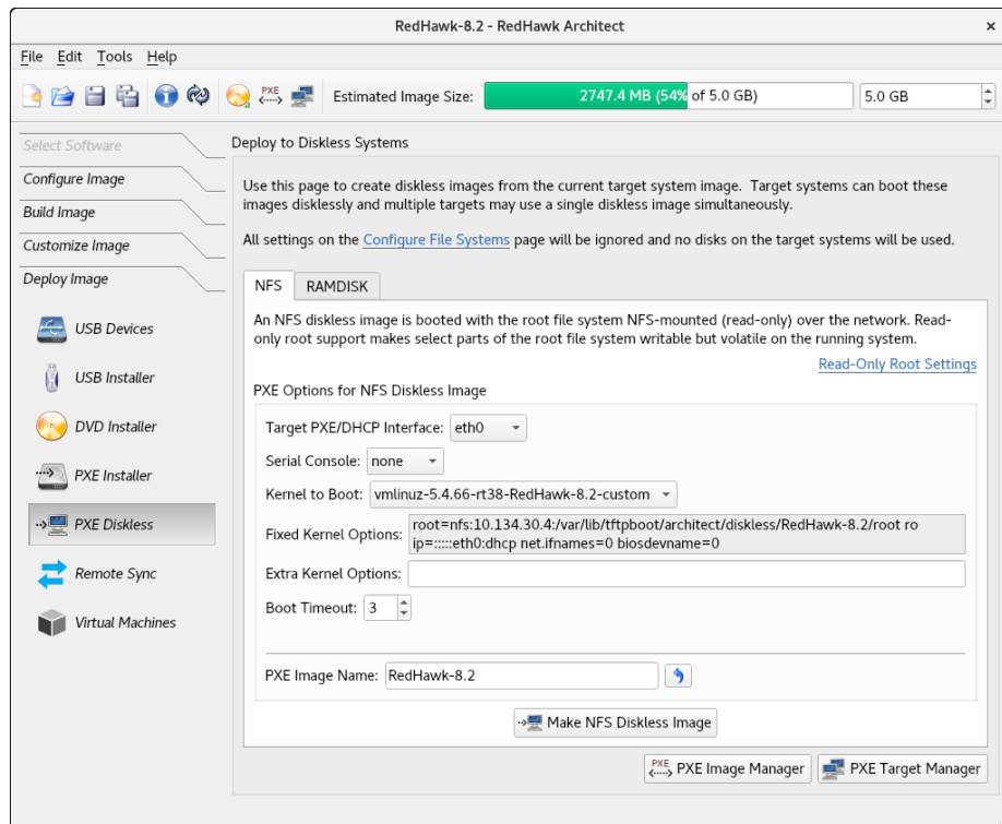
図1-69 PXE NFSディスクレス展開の初期ページ
