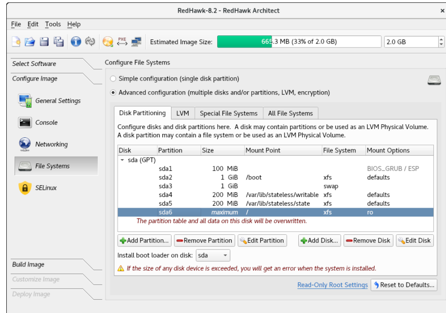
図1-34読み取り専用rootパーティション構想の例
