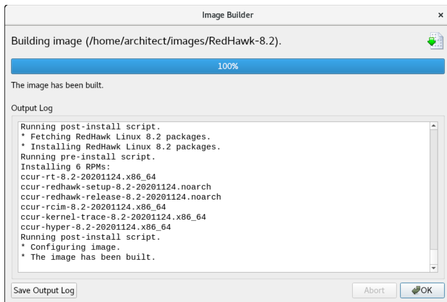
図1-42 RedHawkインストールの状況
