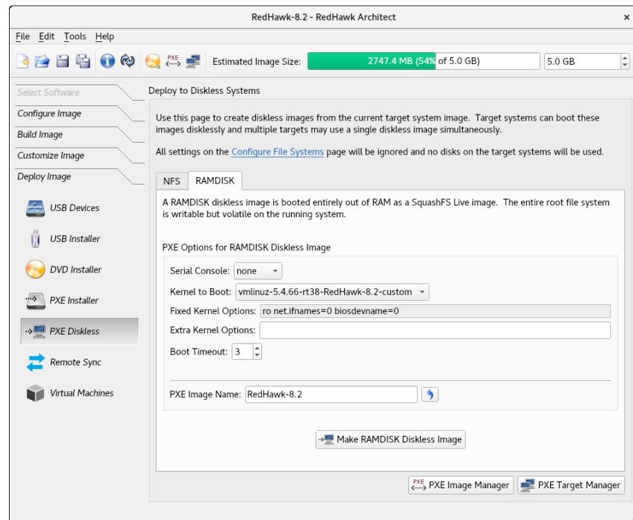
図1-70 PXE RAMDISKディスクレス展開の初期ページ
