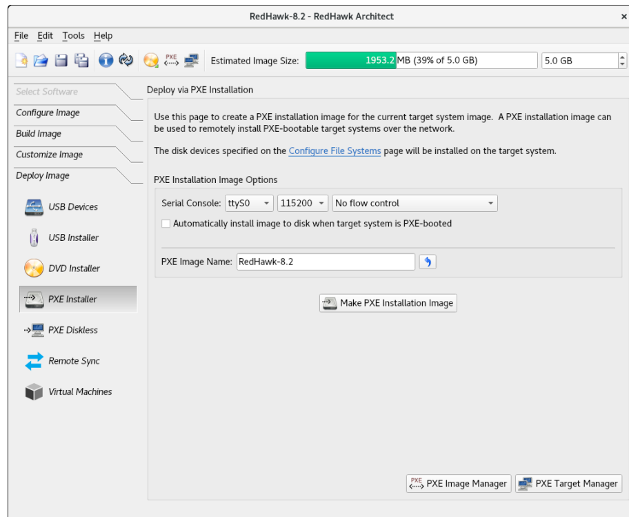
図1-67 Deploy via PXE Installationページ
