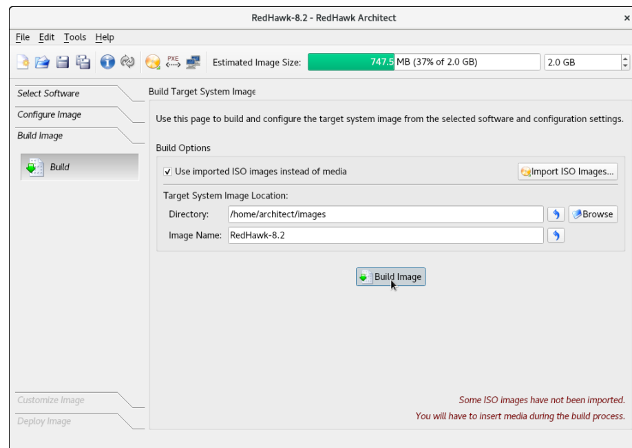
図1-38 Build Imageページ
