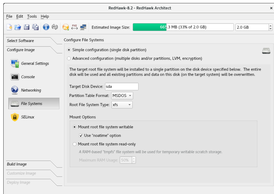
図1-21 File System構成ページ
