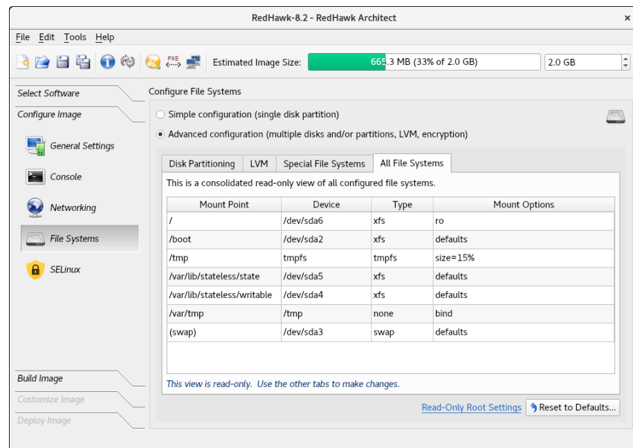
図1-36 全ファイル・システム・リストの例
