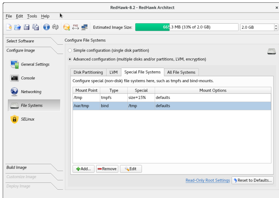
図1-35 特殊ファイル・システムページのエントリー例
