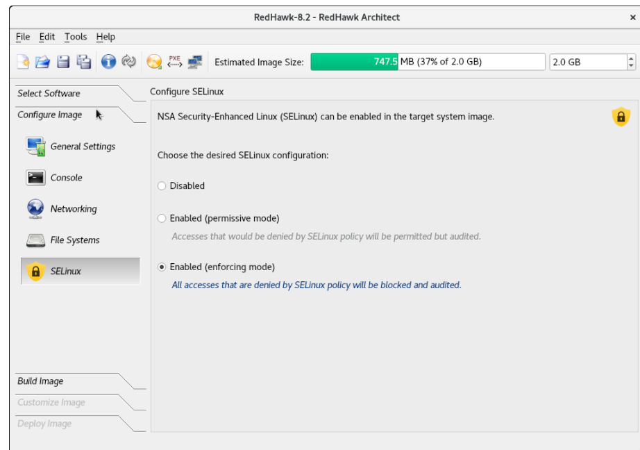
図1-37 SELinuxを強制モードで有効化
