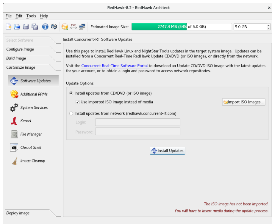
図1-43 Software Updatesページ
