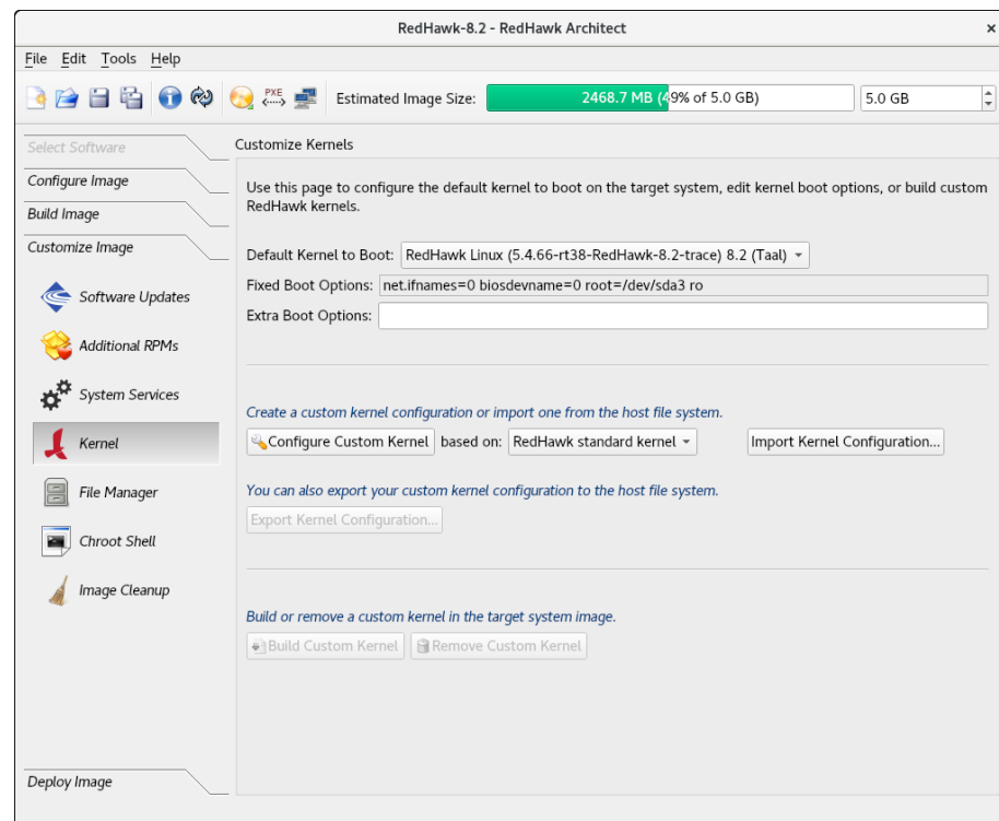
図1-47 Customize Kernelsページ
