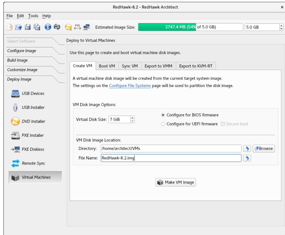
図1-80 Deploy to Virtual Machineページ
