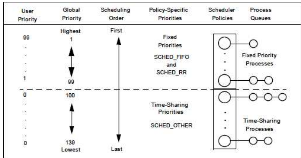
図4-1 スケジューラ
