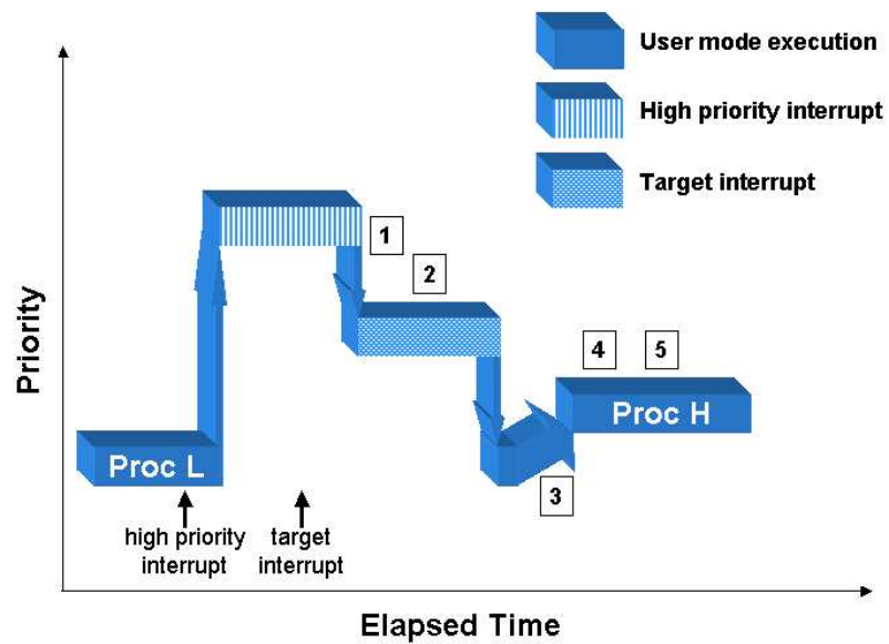
図2-3 高優先度割り込みによるプロセス・ディスパッチ・レイテンシーへの影響
