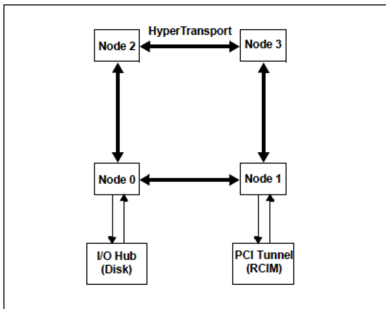
図2-7 クアッドOpteronのI/Oスループット・レイアウト
