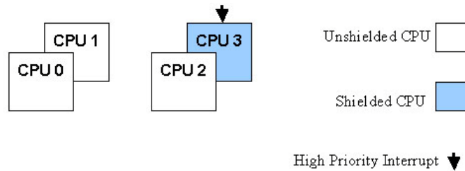
図2-10 ハイパースレッドのシールドリング
