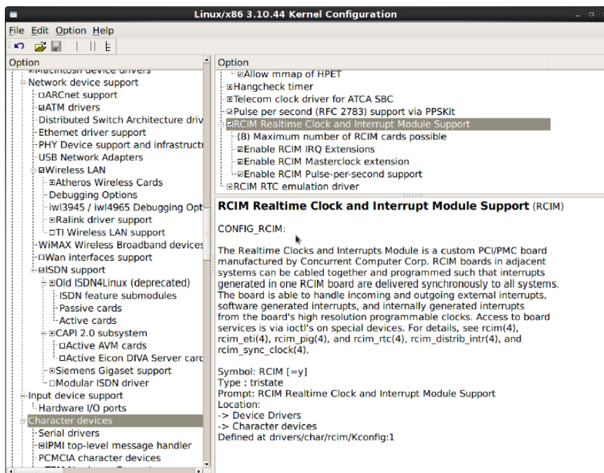
画面11-1 カーネル構成GUI
