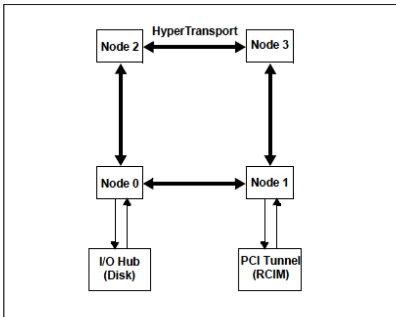
図2-7 クラウドOpteronのI/Oスループット・レイアウト
