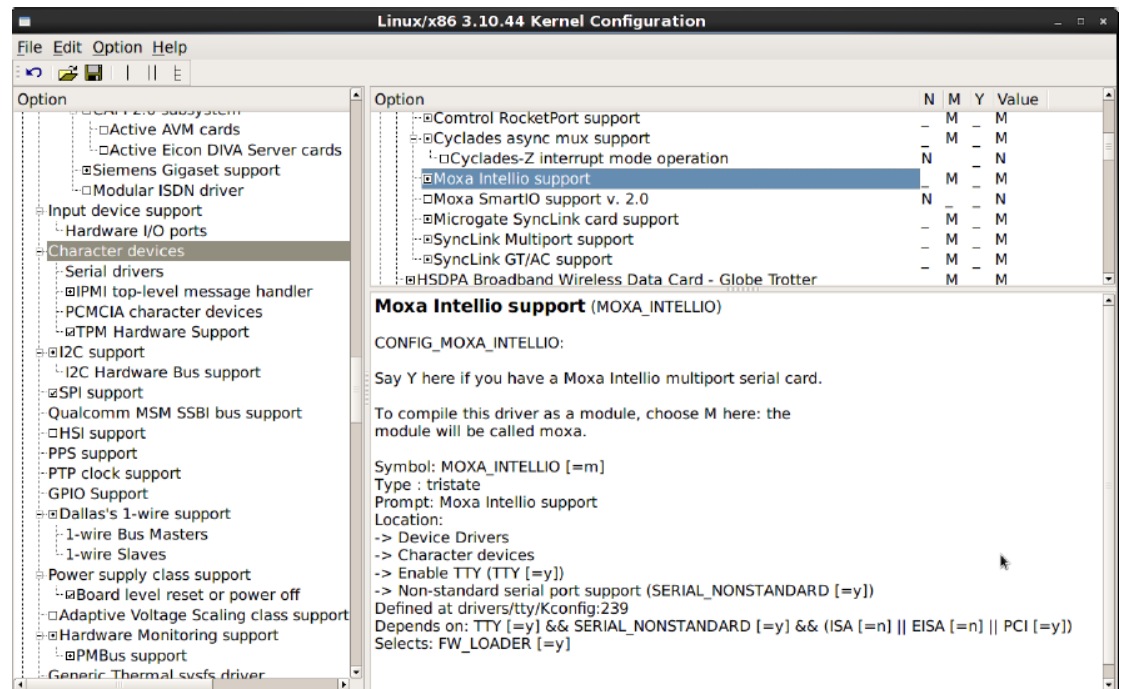
画面11-2 カーネル構成GUIでシリアル・カード・サポートの追加
